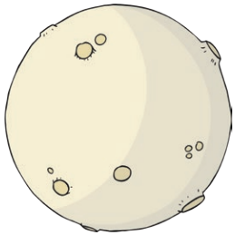
Moon
