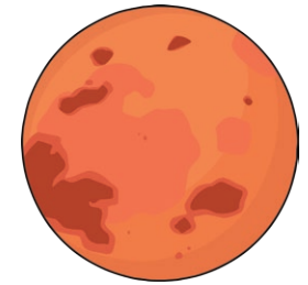
Mars
